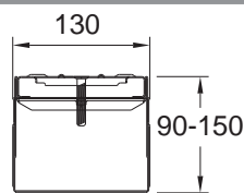
MEATEC 130 výškově nastavitelný 90 mm – 150 mm
