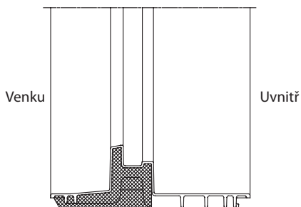
Řez profilem okenní zárubně Komfort, plně tepelně izolované
