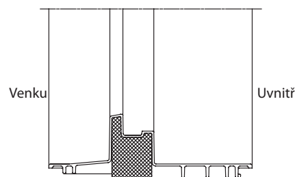
Řez profilem částečně tepelně izolované okenní zárubně
