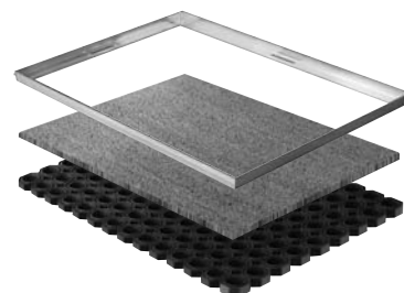
Hliníkový rám, kokosová rohožka, gumová rohožka
